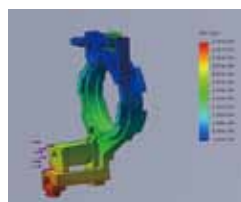
強度解析で耐久性を損なわずにレンズユニットを小型化
